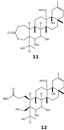
FIGURA 2 (Página anterior y esta). Representaciones esquemáticas de las estructuras químicas de las galphiminas.
